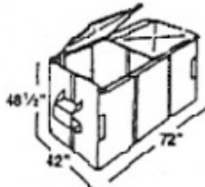
3 Yd. Container
