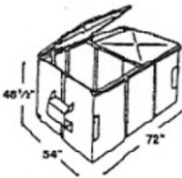
4 Yd. Container
